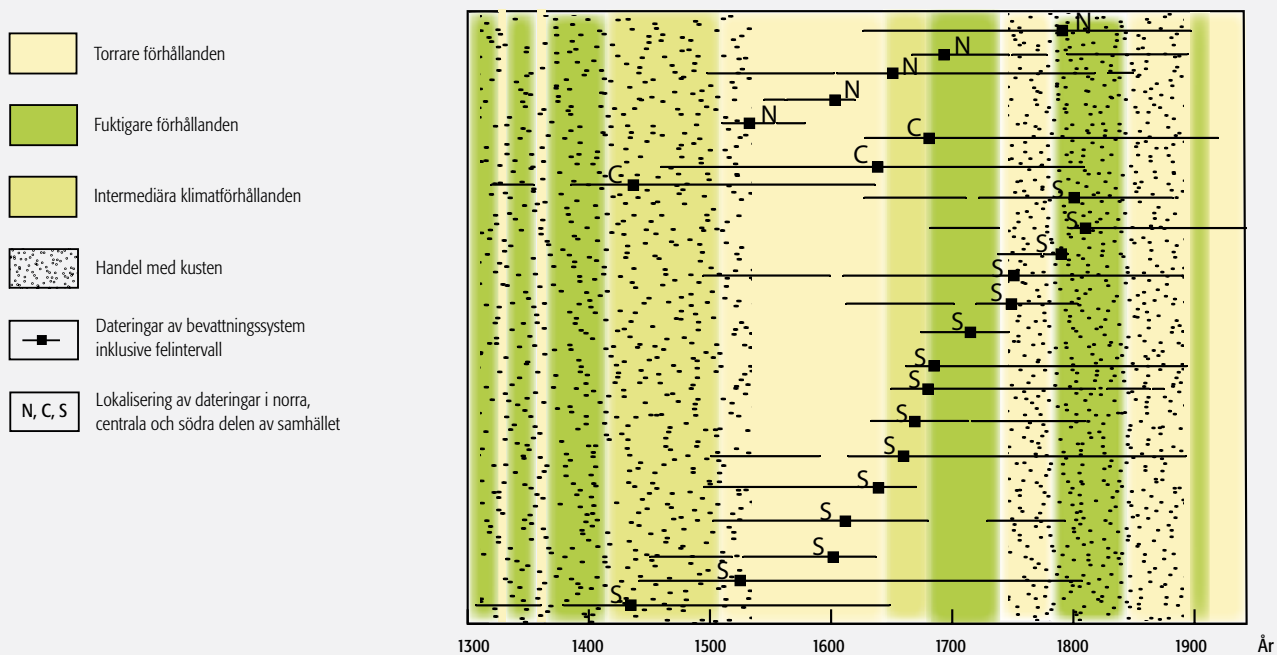
Figur 3. Klimatförhållanden i norra Tanzania de senaste 700 åren. Skiftningarna från grönt till gult speglar växlingar mellan fuktigare och torrare förhållanden. Dateringarna visar under vilket tidsintervall det fossila bevattningssystemet var aktivt, och de rastrerade ytorerna anger när det pågick en aktiv handel mellan Swahilikusten och Östafrikas inland.
