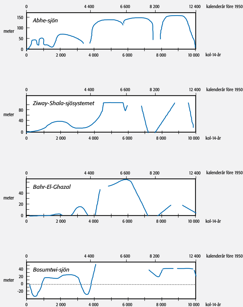
Figur 1. Vattenståndet i sjöar i Etiopien (Abhe, Ziway-Shala), Tchad (Bahr-el-Ghazal) och Ghana (Bosumtwi) under de senaste 12 000 åren. Dateringar görs med den så kallade kol-14-metoden och åldrarna omvandlas därefter till kalenderår före 1950. Åldern noll på diagrammets x-axel betyder alltså år 1950.
